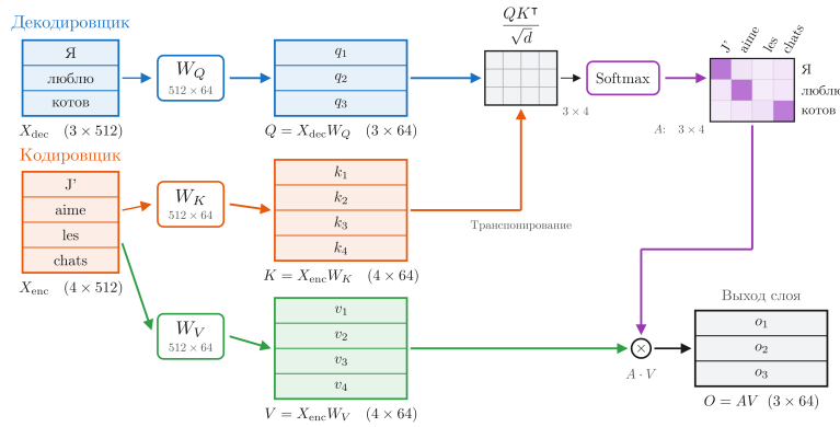
Рис. 21: Схема перекрестного внимания.
