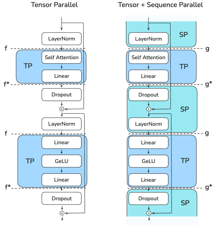
Рис. 56: TP+SP параллелизм. Взято из Ultra-Scale Playbook.
