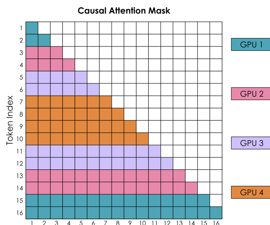
Рис. 59: Распределяем токены так, чтобы выровнять нагрузку на ранги. Взято из Ultra-Scale Playbook.
