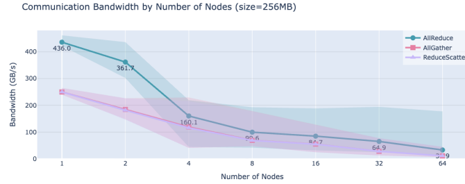
Рис. 60: Пропускная способность межнодовой коммуникации в зависимости от количества нод. Взято из Ultra-Scale Playbook.
