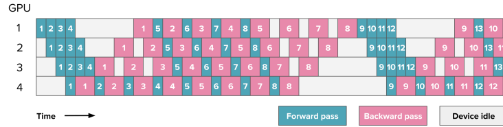
Рис. 63: 1F1B. Взято из Ultra-Scale Playbook.
