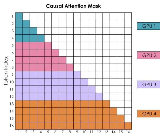
Рис. 58: Разделение ‘зон ответственности’ вычисления матрицы внимания между рангами при контекстном параллелизме. Взято из Ultra-Scale Playbook.
