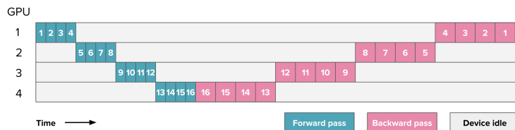
Рис. 61: AFAB. Взято из Ultra-Scale Playbook.
