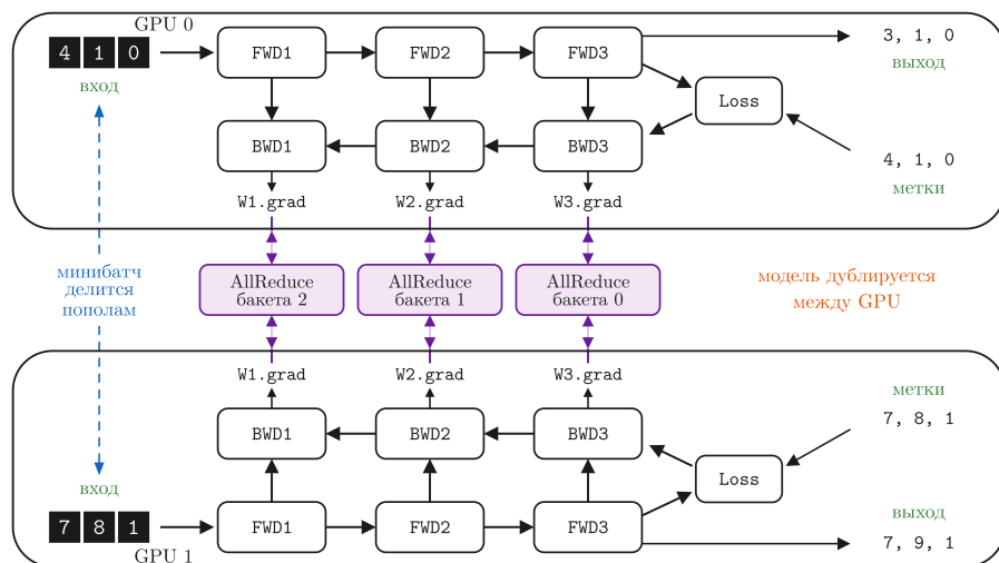
Рис. 47: Схема распределенного параллелизма данных между двумя девайсами с разделением AllReduce градиентов по бакетам.
