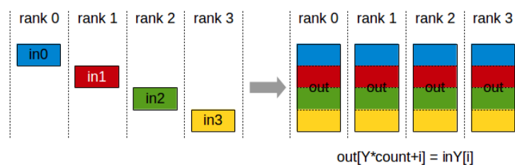
Рис. 39: Схема AllGather.
