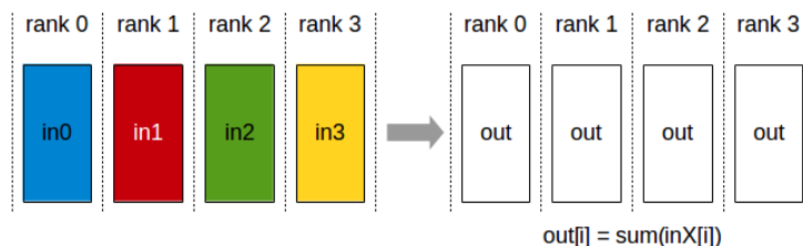
Рис. 37: Схема AllReduce.
