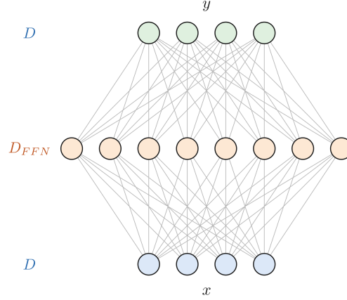
Рис. 22: Схема FFN-слоя.
