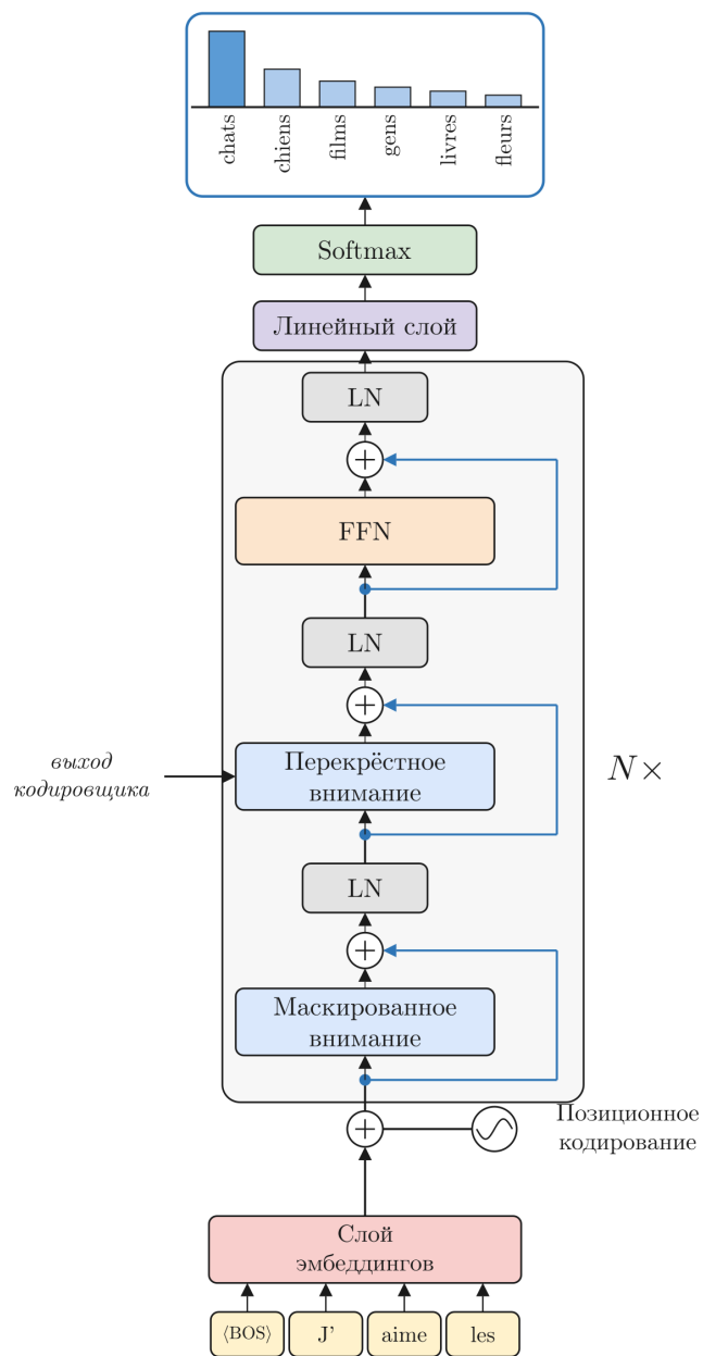
Рис. 24: Схема трансформера-декодировщика.
