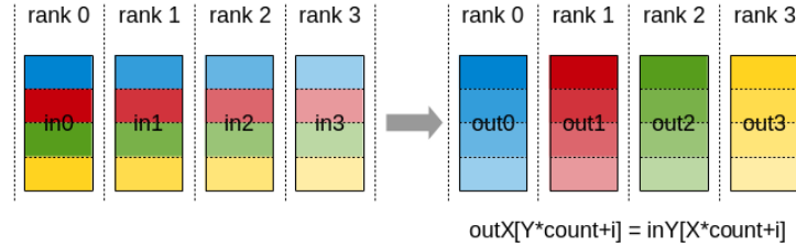
Рис. 42: Схема AlltoAll.
