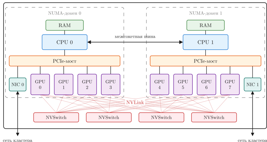
Рис. 33: Схема ноды.
