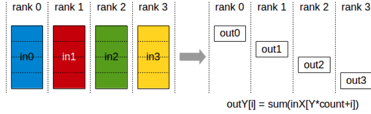
Рис. 41: Схема ReduceScatter.
