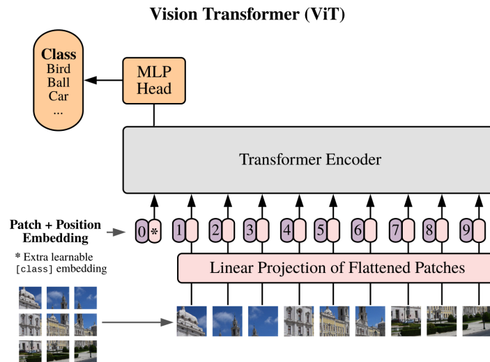
Рис. 26: Архитектура ViT. Взято из оригинальной статьи “An Image is Worth 16x16 Words”.
