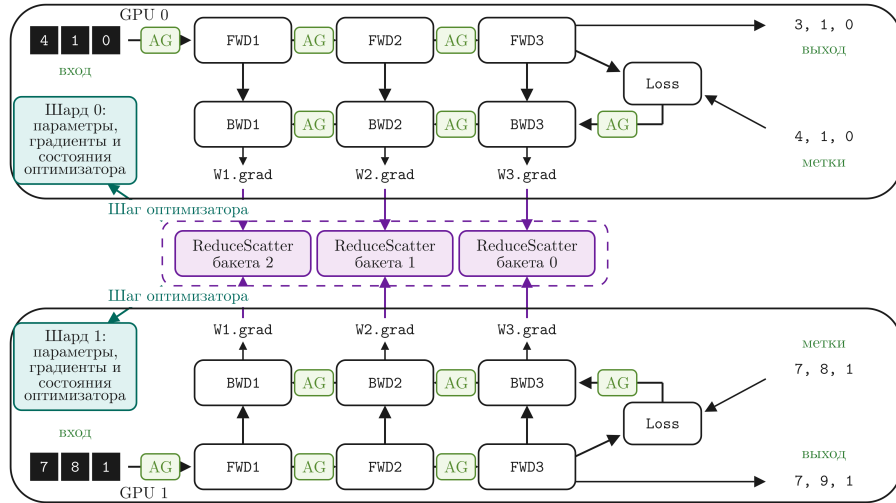
Рис. 51: FSDP (ZeRO-3). Параметры, градиенты и состояния оптимизатора шардируются между рангами. AG — AllGather коммуникация.
