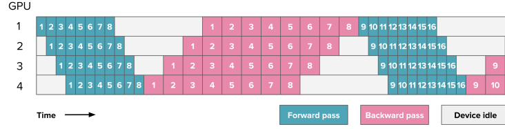
Рис. 62: AFAB по микробатчам. Взято из Ultra-Scale Playbook.
