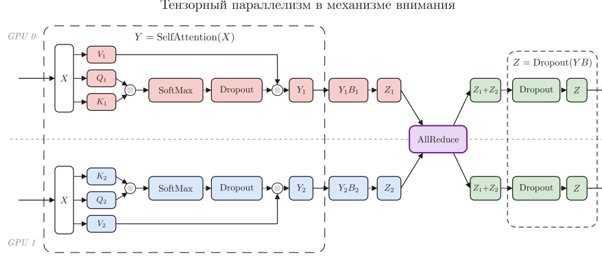
Рис. 55: Применение тензорного параллелизма при вычислении многоглавого внимания.
