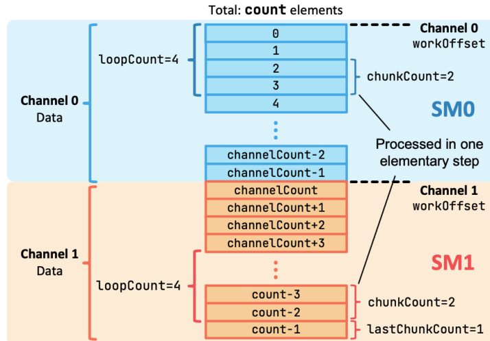
Рис. 43: Визуализация стратегии разделения данных NCCL между каналами.
