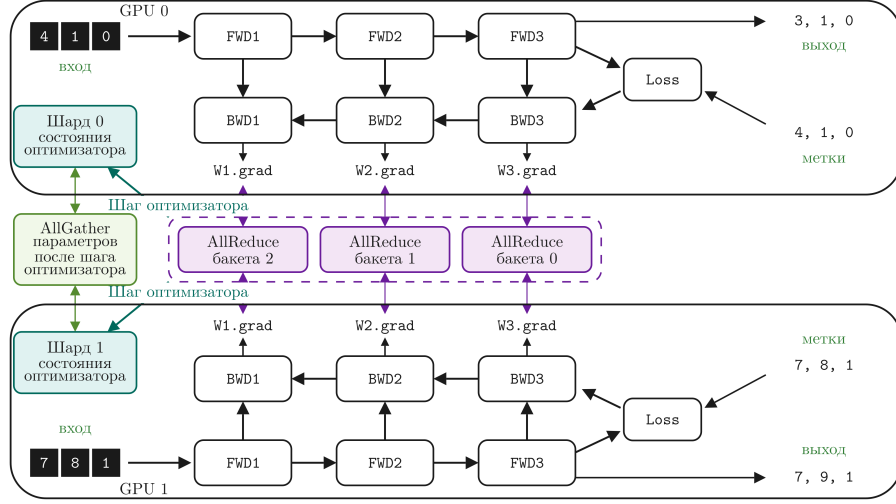
Рис. 49: ZeRO-1. Состояния оптимизатора шардируются между рангами, а параметры и градиенты реплицируются.
