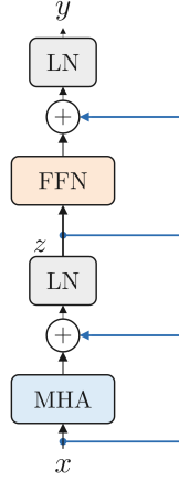
Рис. 23: Схема остаточных связей.
