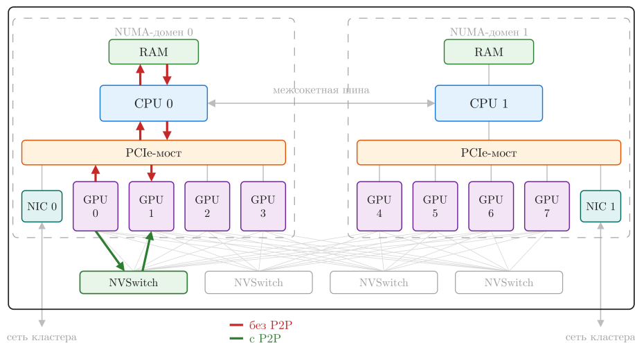
Рис. 34: Схема P2P-связи между GPU.
