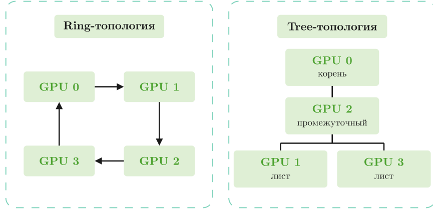
Рис. 44: Схемы алгоритма коммуникации по кольцу (слева) и коммуникации по дереву (справа).
