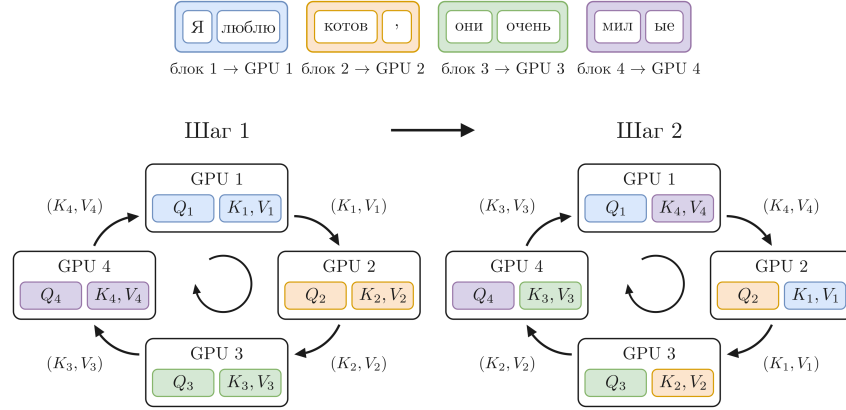
Рис. 57: Схема кольцевого внимания.
