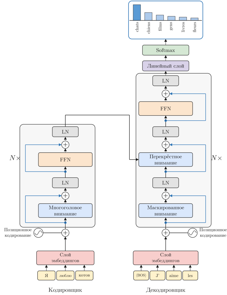
Рис. 25: Архитектура трансформера кодировщика-декодировщика, взято из оригинальной статьи "Attention is all you need".
