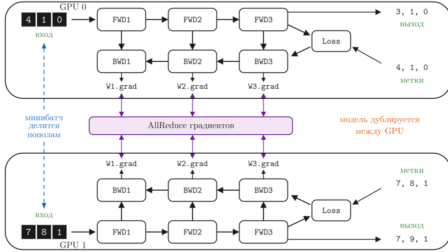
Рис. 46: Схема распределенного параллелизма данных между двумя девайсами. FWD — этап прямого распространения, BWD — этап обратного распространения.
