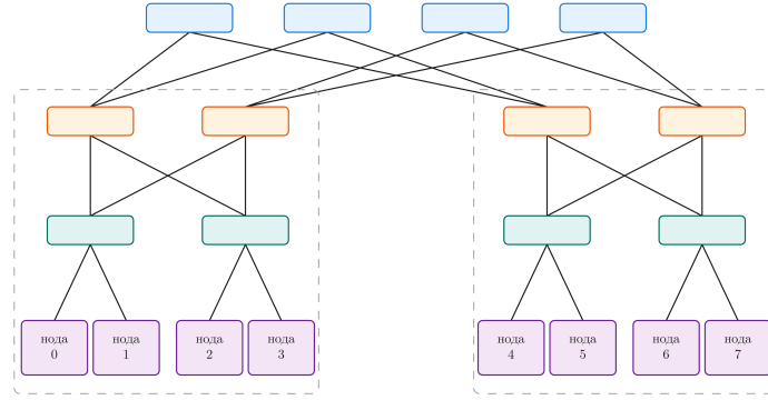
Рис. 36: Схема fat-tree топологии.
