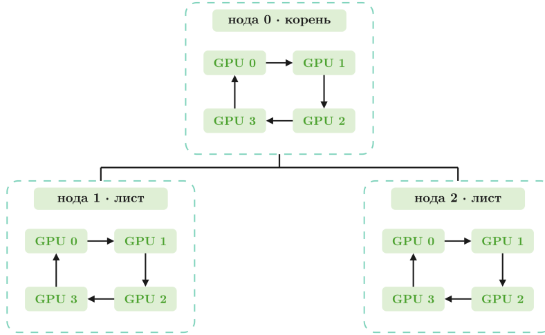
Рис. 45: Схема коммуникации в иерархической топологии. Внутри нод используется кольцевой алгоритм, а между нодами — древовидный.
