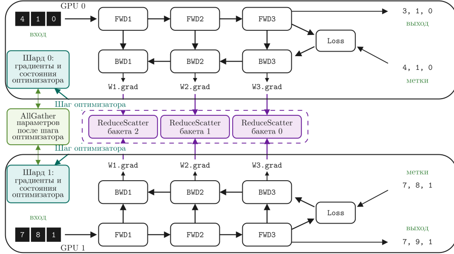
Рис. 50: ZeRO-2. Градиенты и состояния оптимизатора шардируются между рангами, а параметры реплицируются.
