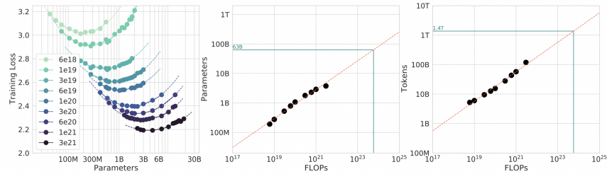
Рис. 67: Анализ IsoFLOPs
