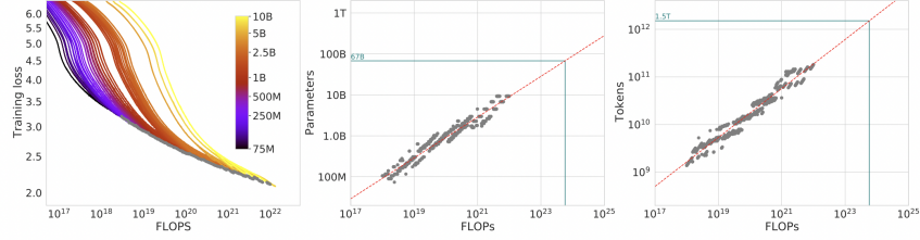
Рис. 66: Минимум объединения кривых
