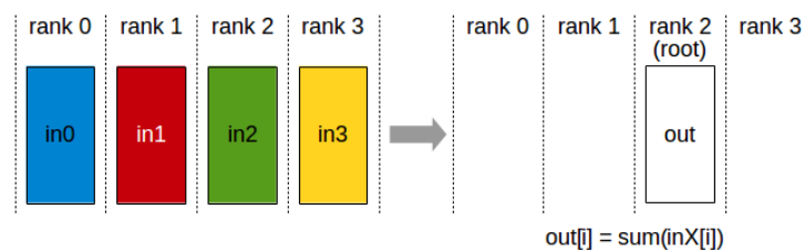
Рис. 40: Схема Reduce.
