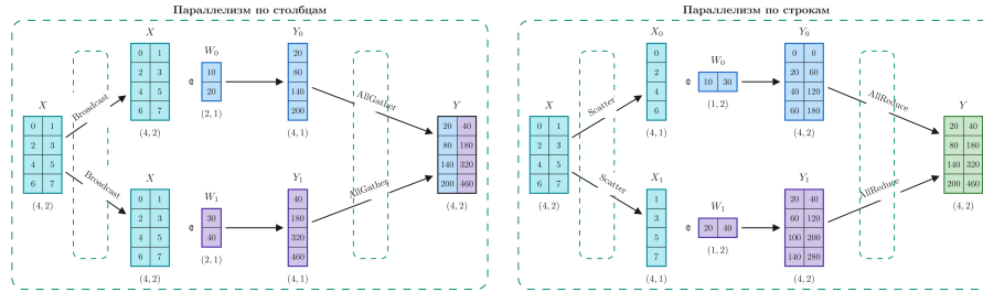
Рис. 53: Схема параллелизма по столбцам (слева) и по строкам (справа).
