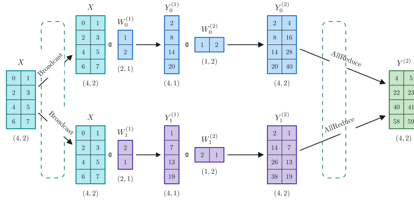
Рис. 54: Схема вычисления FFN-блока с использованием сначала параллелизма по столбцам, а следом — параллелизма по строкам.
