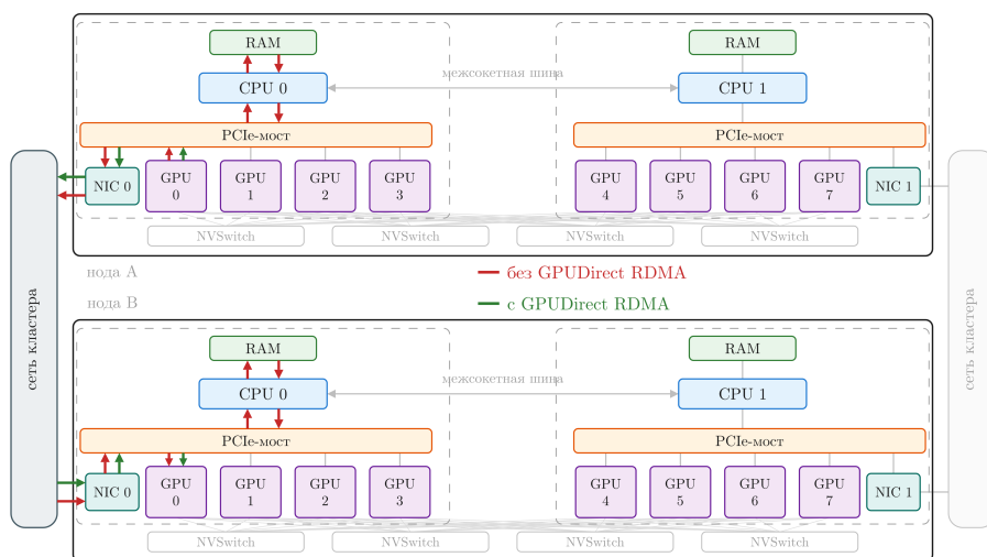
Рис. 35: Схема RDMA-связи между GPU.
